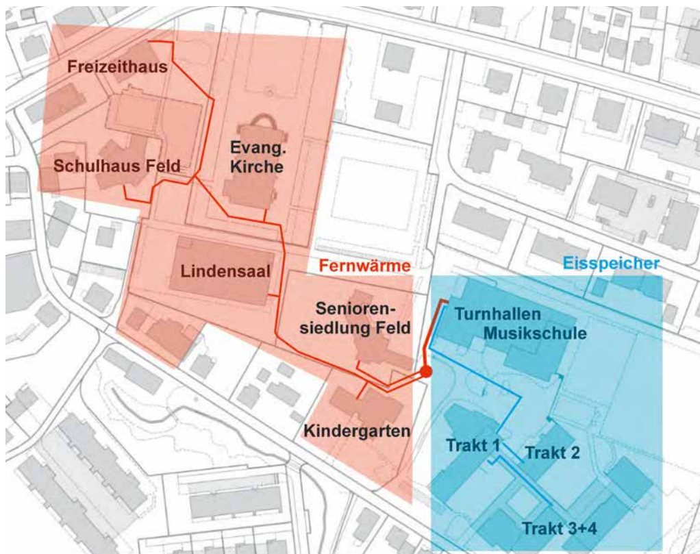
Die neue Aufteilung des Nahwärmeverbunds: Der rote Bereich wird mit Fernwärme beheizt, der blaue mit dem Eisspeicher
