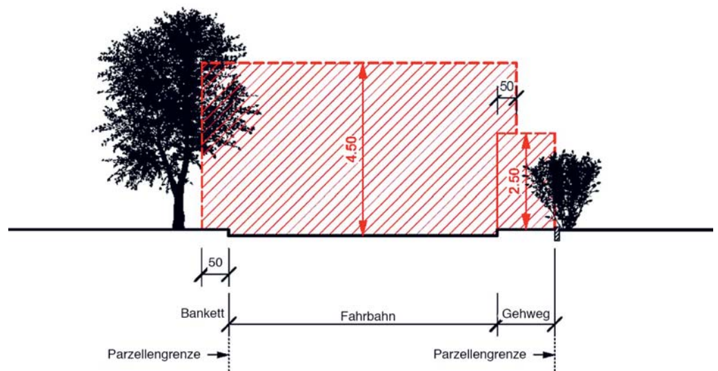
Die schraffierte Fläche ist von überhängenden Ästen und Sträuchern freizuhalten. Die Höhe des Lichtsraums beträgt 4,50m über Verkehrsflächen, die für den Fahrverkehr bestimmt sind, und 2,50m über Verkehrsflächen, die nicht für den Fahrverkehr bestimmt sind.
