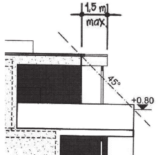
Neue Bestimmungen für Attikageschosse: Dachvorsprünge bei Attikaterassen dürfen maximal 1,50 m betragen.
